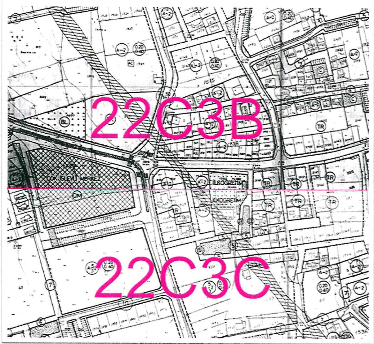
Şekil 3: 1/1000 ölçekli Çeşmealtı Revizyon İmar Planı
